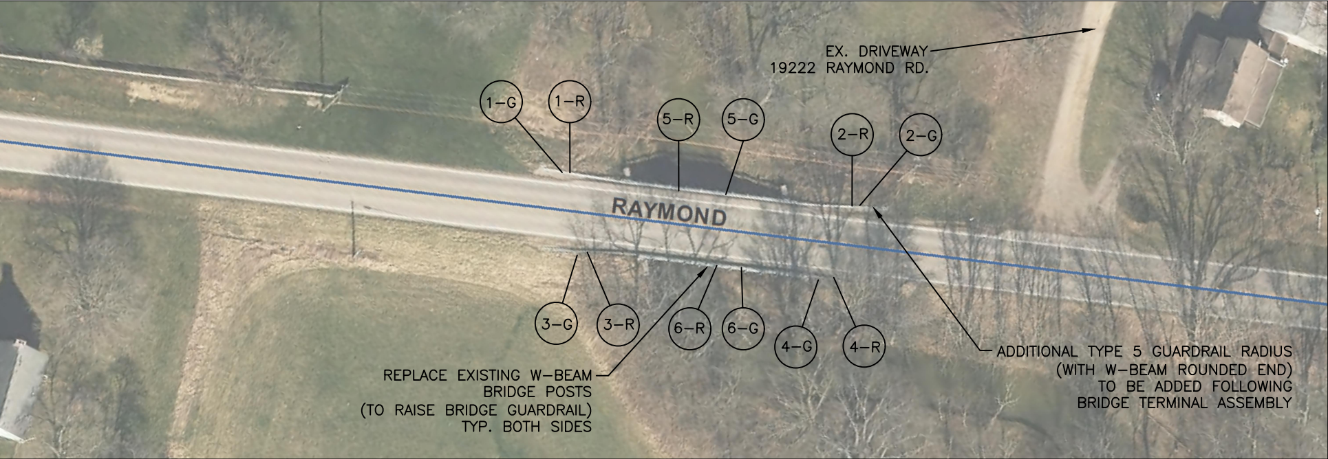
CR 191 – RAYMOND ROAD – MM 5.12 N.T.S.
